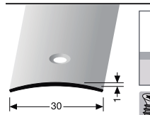
451 mittig versenkt gebohrt
