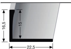
306 U ± 15 mm ungestanzt
